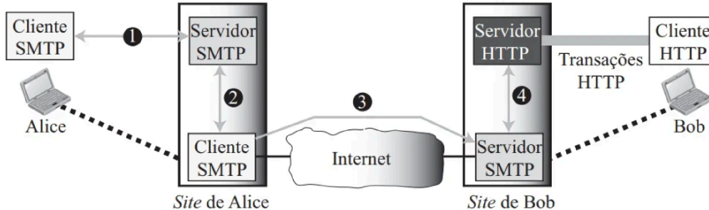
Caso 1: Apenas o destinatário usa HTTP
